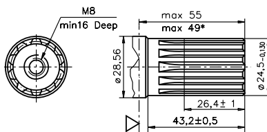
SA - splined, B25x22xh9 DIN 5482 Max. Torque 40 daNm
