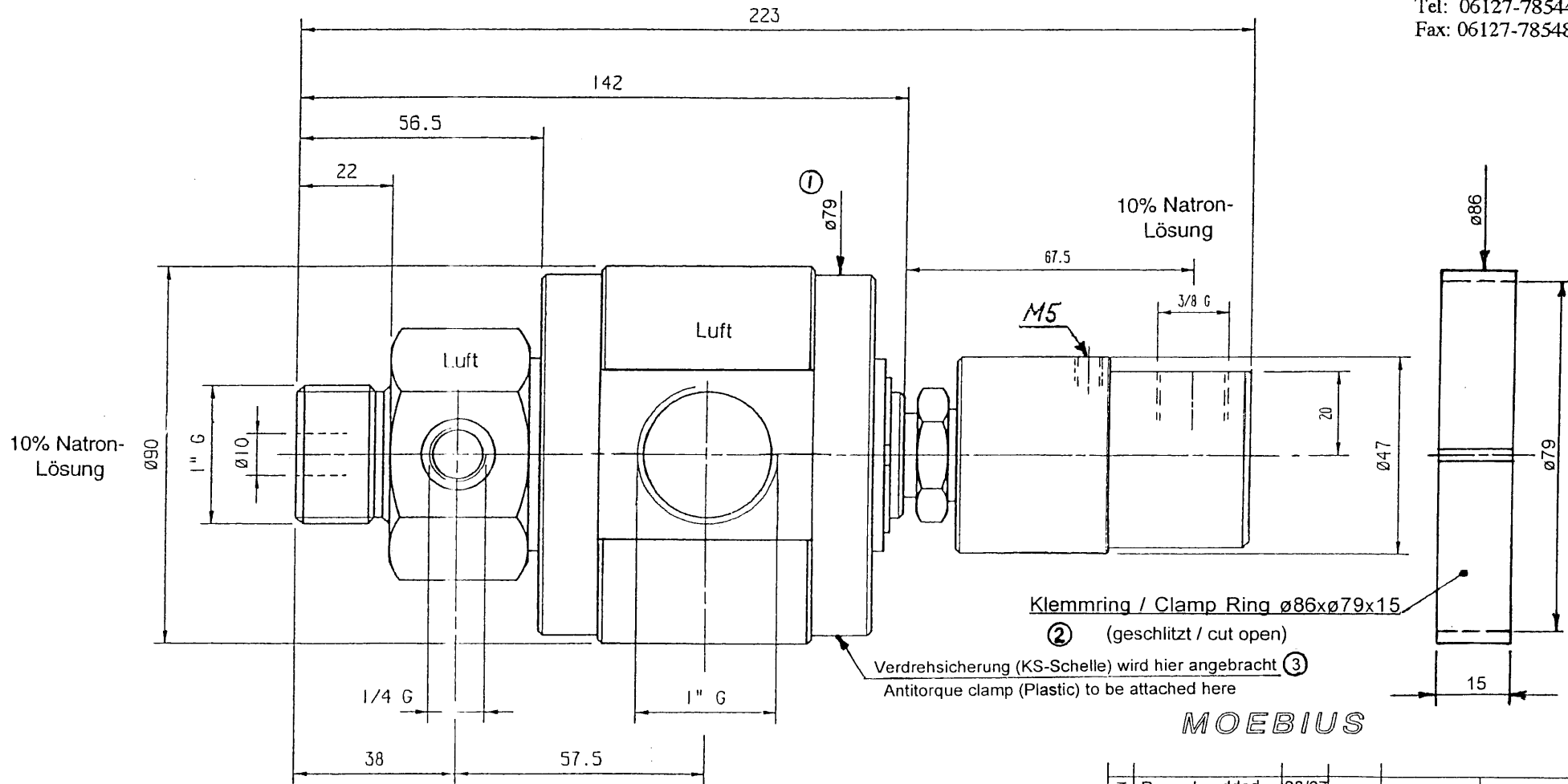
TURIAN Tandem-Drehdurchführung für Luft + 10% Natron-Lösung GSN 25T-SsM5
